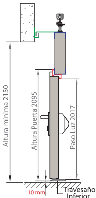
Vista Sección
